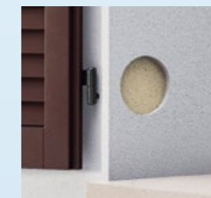
Particolare bocchetto in purenit inserito all'interno alla spalla per fissaggio cardini.
